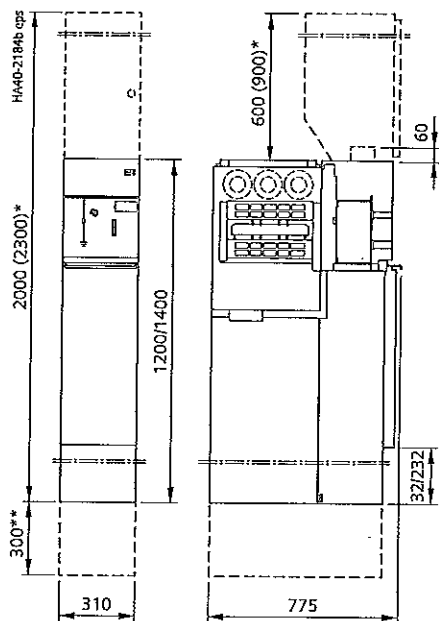
Шинозаземителен панел тип Е
