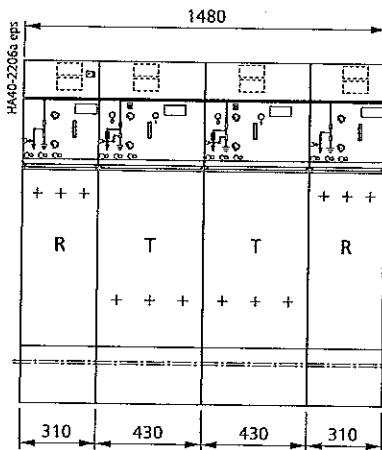
Схема RTTR
