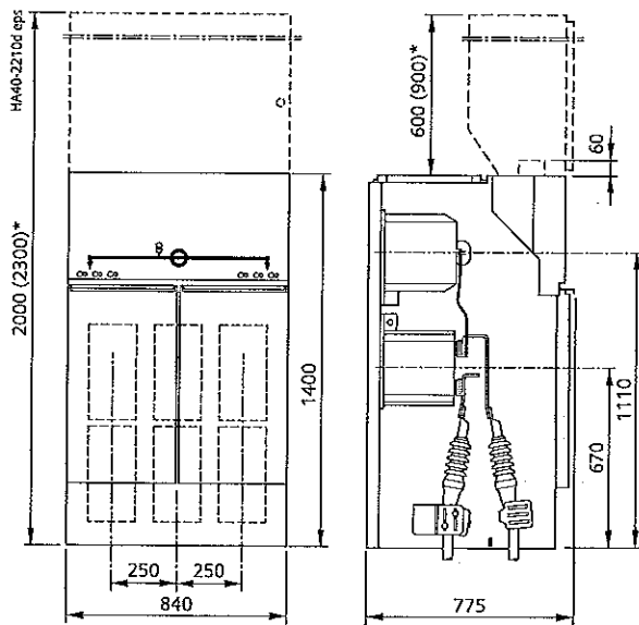
Присъединение: кабел-кабел
