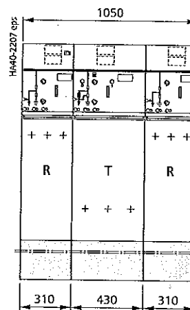
Схема RTR
