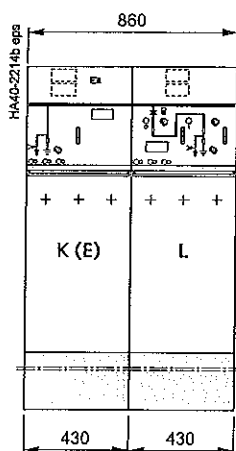
Схема K(E)L
