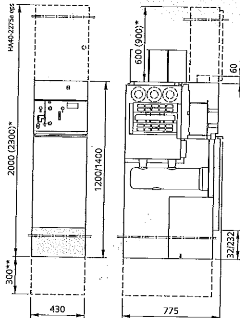
Панел мерене тип M(430) с разедияем напреженов трансформатор с предпазители на първичната страна
