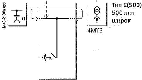
Панел заземяване на шините
