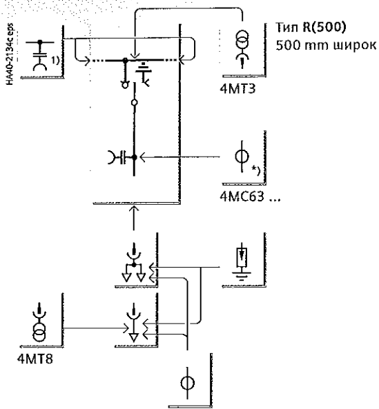
Извод вход-изход
