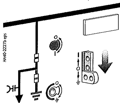
Освобождаване за действие на заземяващия нож
