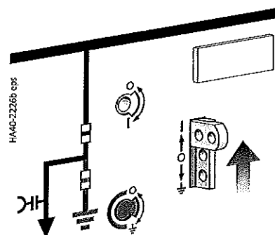
Освобождаване за действие на разединителя
