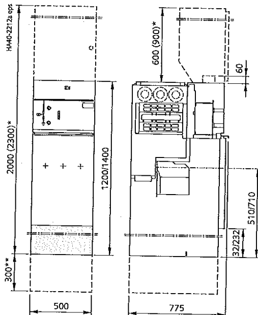
Панел мерене тип M(500) с разедияем напреженов трансформатор
