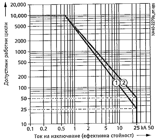
Номинален ток на изключване при късо съединение 25 kA
