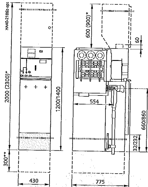
Кабелен извод тип K(E) със заземителен нож с мигновено пружинно действие
