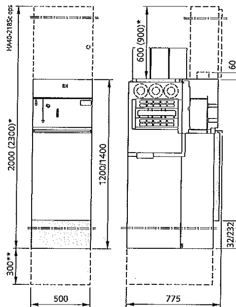
Шинозаземителен панел тип Е(500) с напрежен трансформатор
